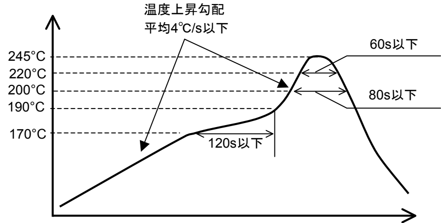
図-4 はんだリフロー条件
