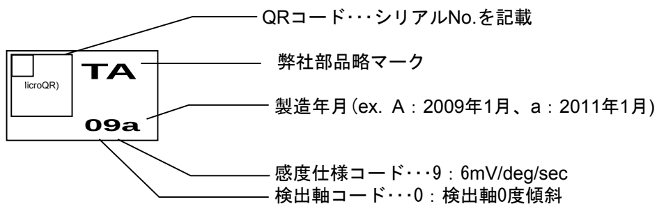
図-2 捺印図
