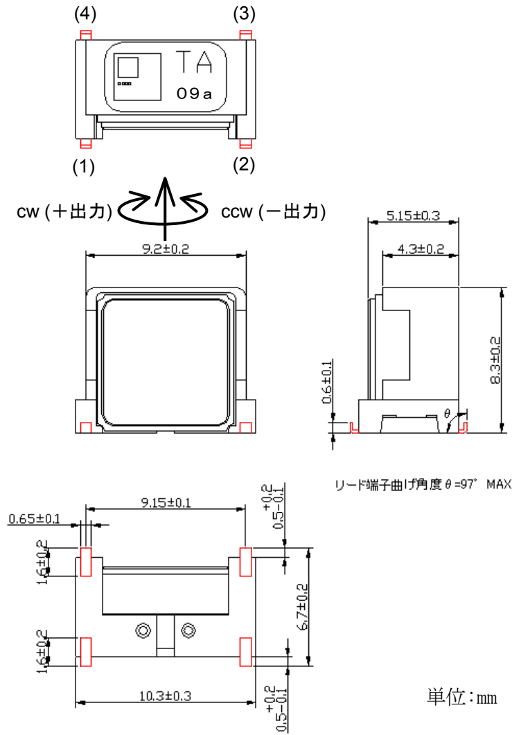
図-1 製品図
